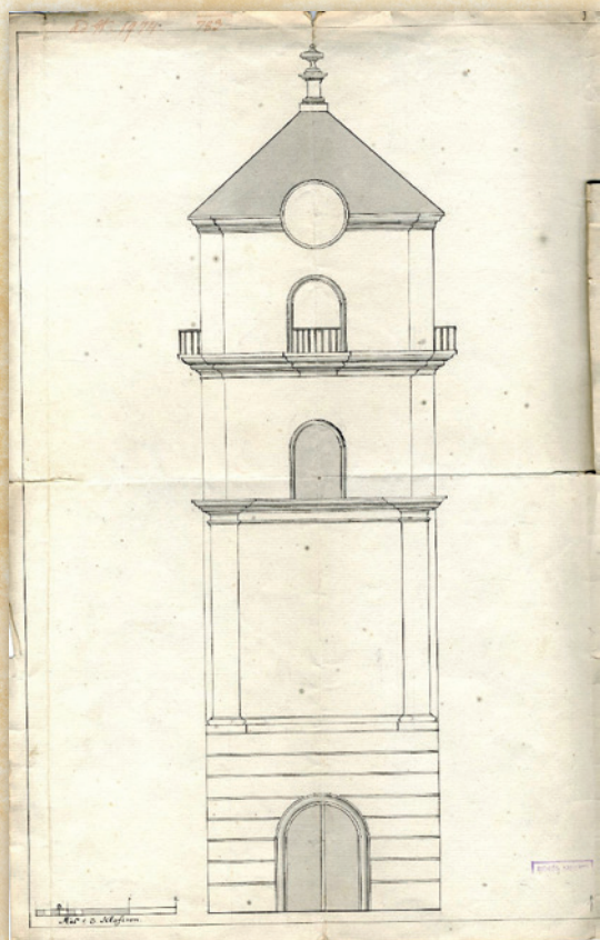
A békéscsabai evangélikus templom tornyának tervrajza, 1782
