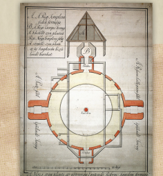
A debreceni Református Nagytemplom Felirátja Mihály építész által tervezett - végül még nem valósult - kerek templom tervezés alaprajza, 1803. MNL. FM. V. 11. B. 10.
